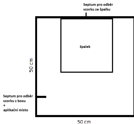
Obrázek 3.4.2: Nákres fumigačního boxu s dřevěným blokem v průběhu testu.
